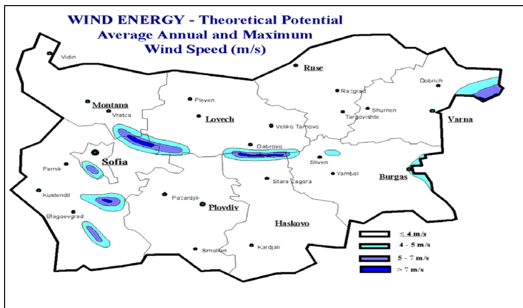
фиг.5 Картохема на ветровия потенциал в България
