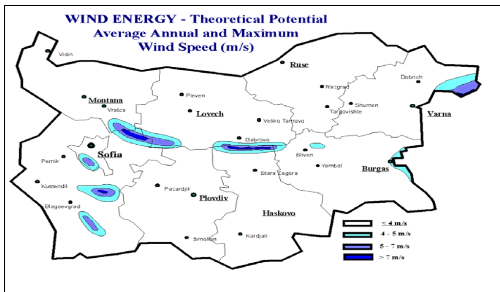
фиг.5 Картосхема на ветровия потенциал в България
